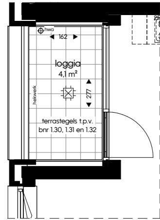
1e verdieping - bnr 1.30, 1.31 en 1.32
